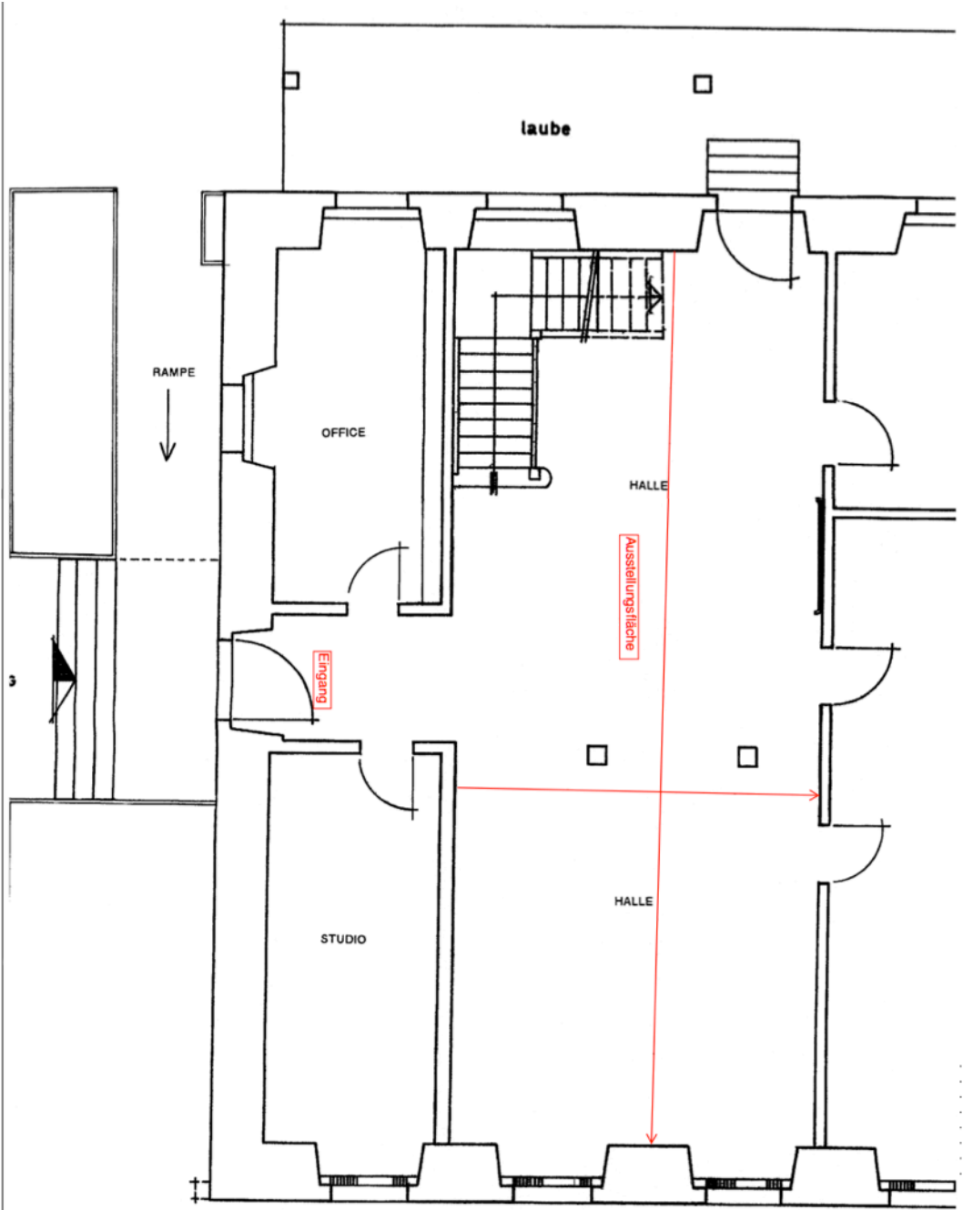
ERDGESCHOSS
